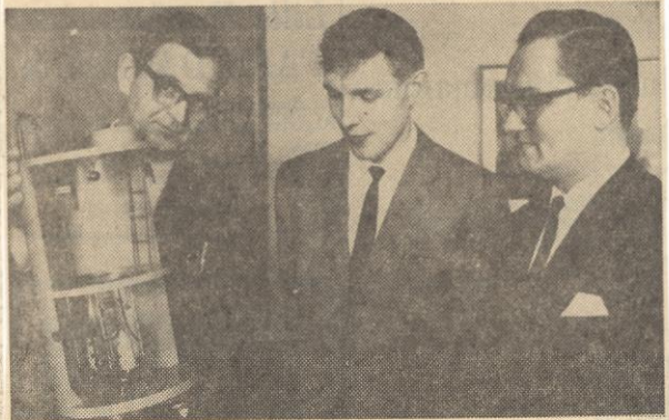
Fabrikör Helmuth Fischer demonstrerar en modell av genomskärningen av en avloppspumpstation utrustad med Fischer pumpar. Längst till höger ingenjör Pertti Kuortti och i mitten Tulifas Norrlands AB:s driftsingenjör Thomas Lindsten.
